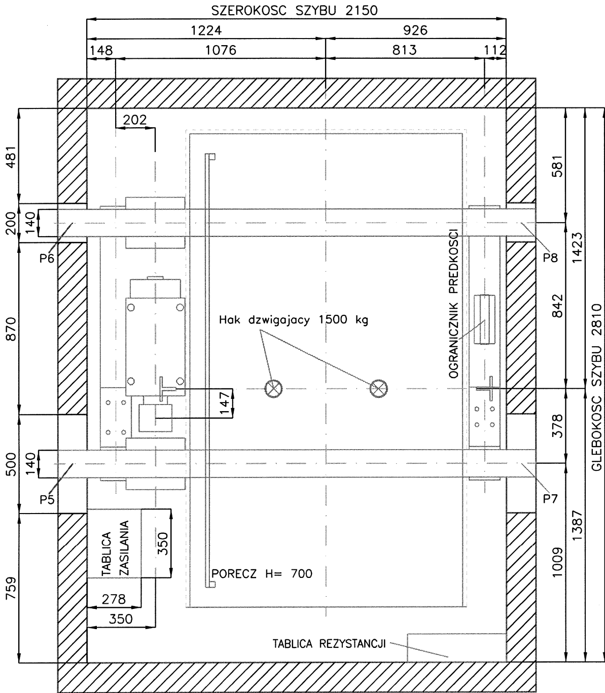
RZUT MASZYNY
